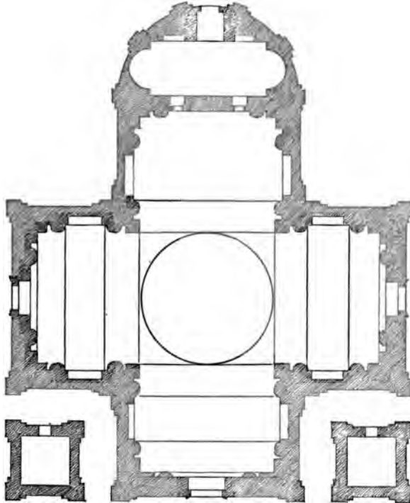
FIG. 37. — Plan of San Biagio.
